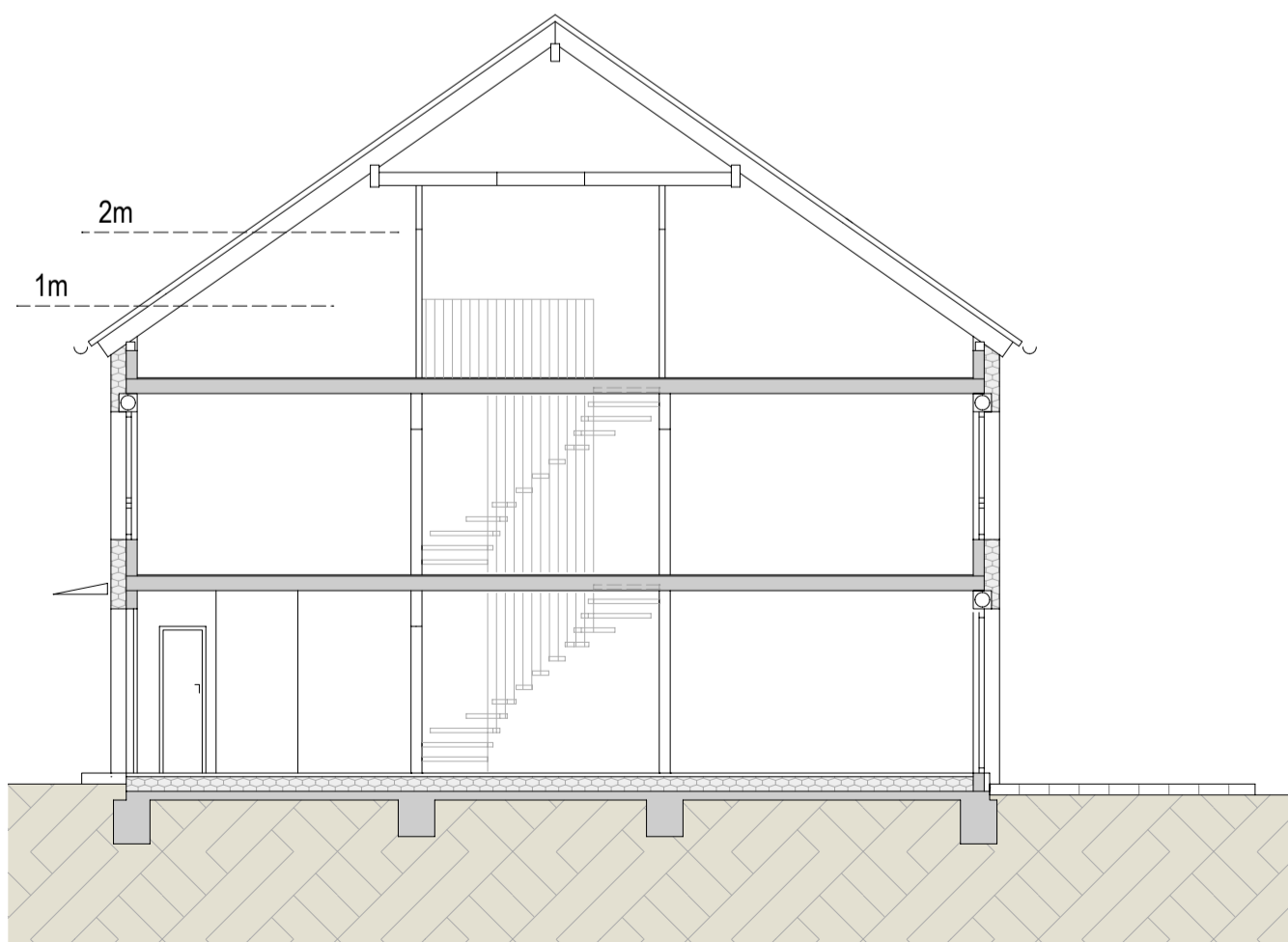
SCHNITT
